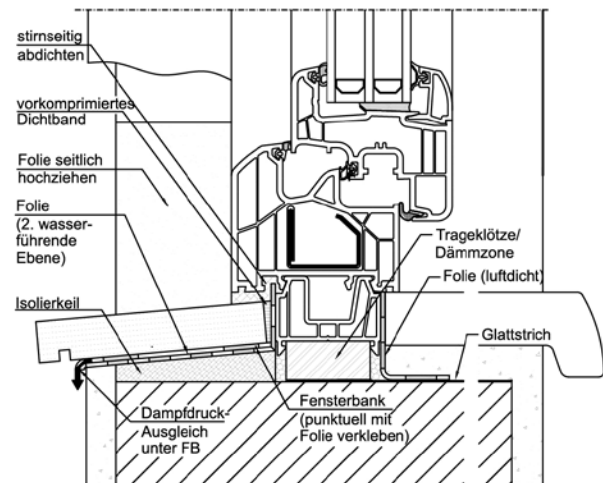
Unterer Anschluss mit Stein-Fensterbank.
