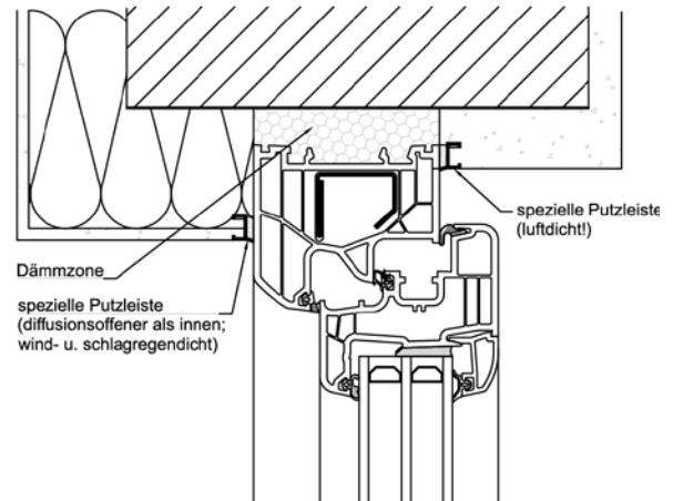
Oberer Anschluss mit Vollwärmeschutz.
